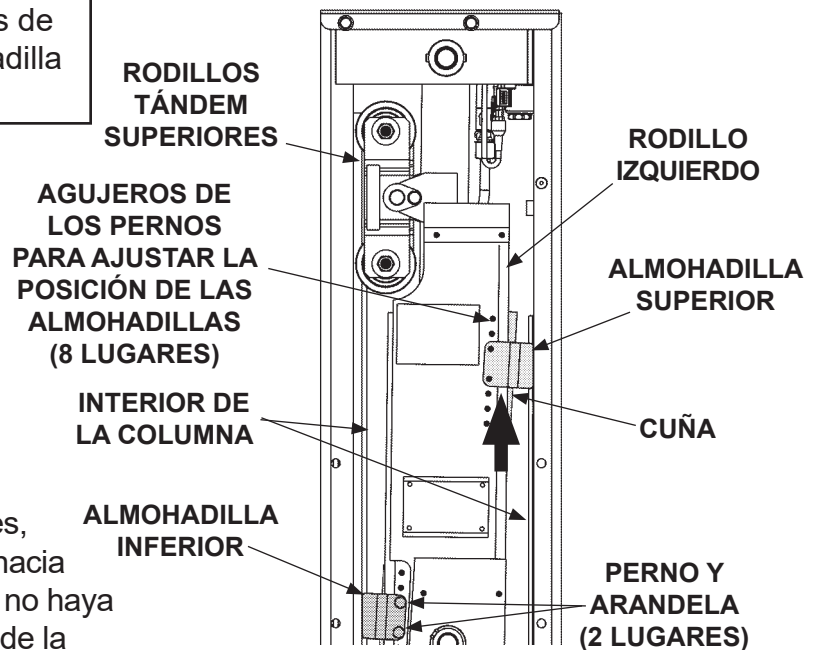
ATORNILLAR LA ALMOHADILLA INFERIOR Y AJUSTAR LA ALMOHADILLA SUPERIOR FIG. 88-2
