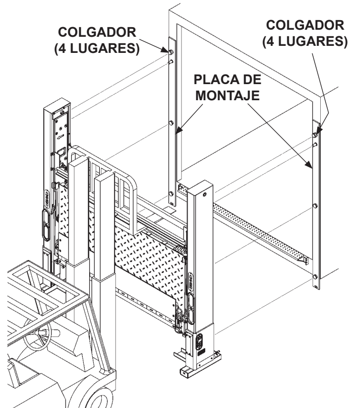
COLGAR EL ELEVADOR FIG. 37-1
