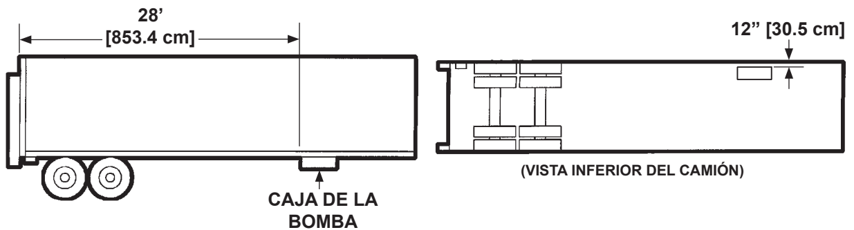
INSTALACIÓN USUAL PARA 28 PIES [853.4 cm] FIG. 42-3
