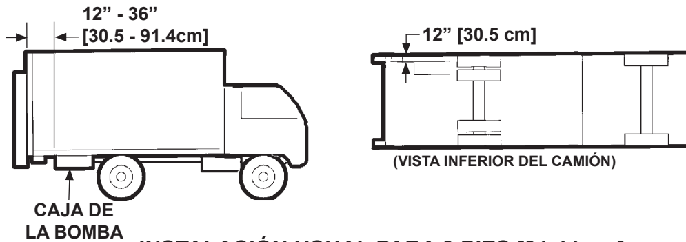
INSTALACIÓN USUAL PARA 3 PIES [91.44 cm] FIG. 41-1
