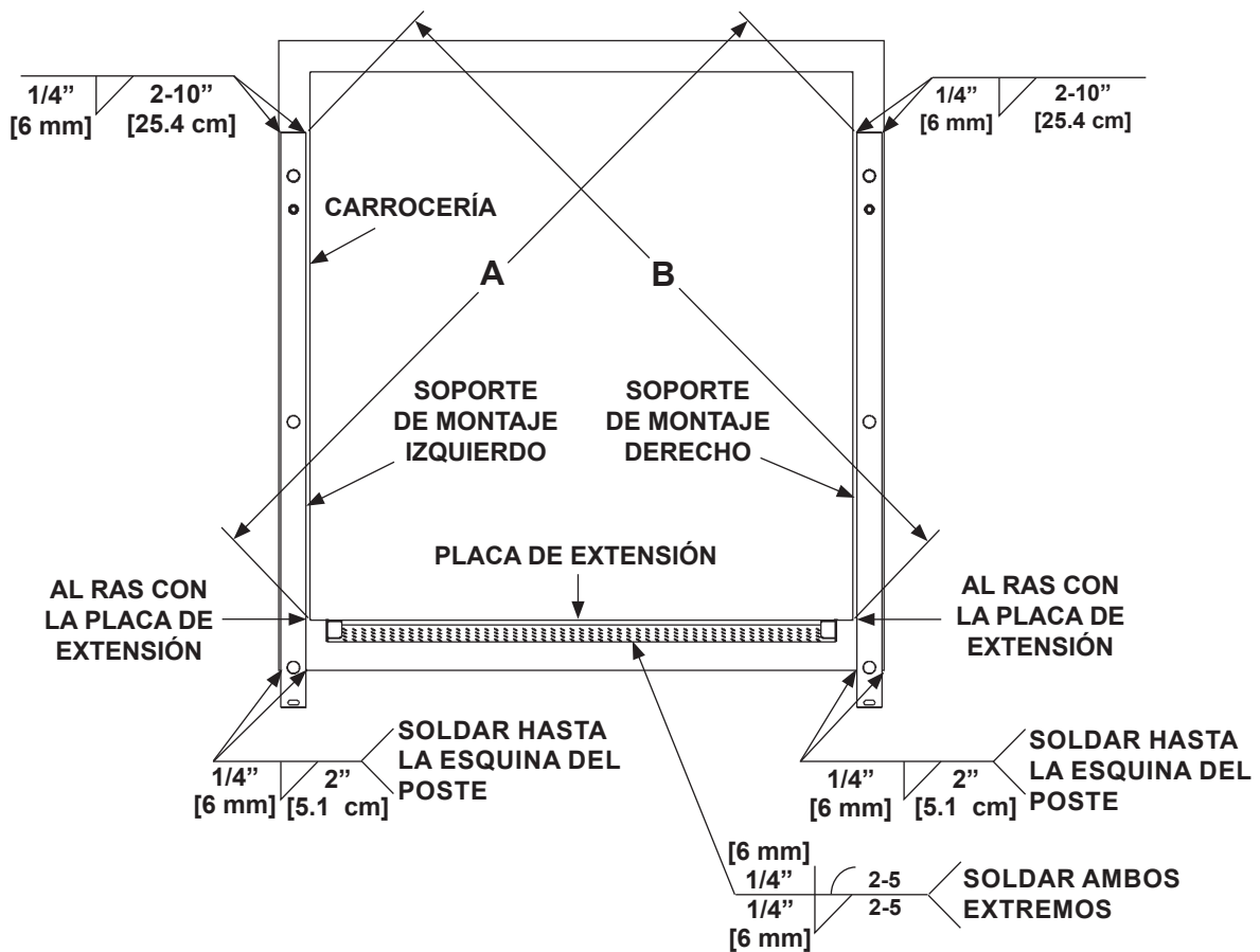
PARTE POSTERIOR DE LA CARROSERÍA DEL VEHÍCULO FIG. 26-1
