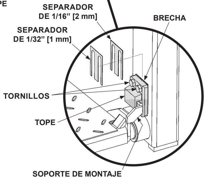
VISTA POSTERIOR DE CORREDERA IZQUIERDA FIG. 84-1A
