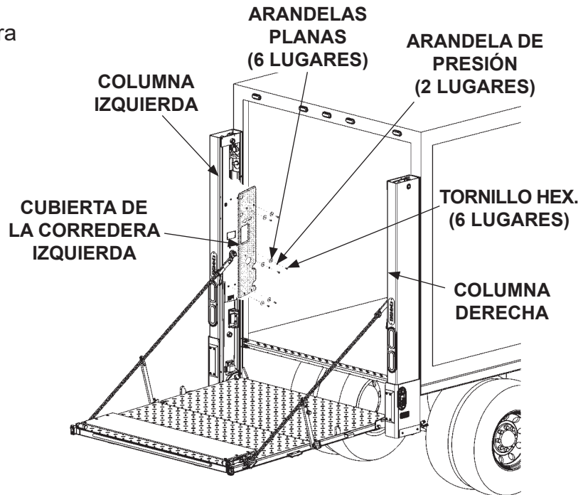
RETIRAR LAS CUBIERTAS DE LAS CORREDERAS FIG. 87-1
