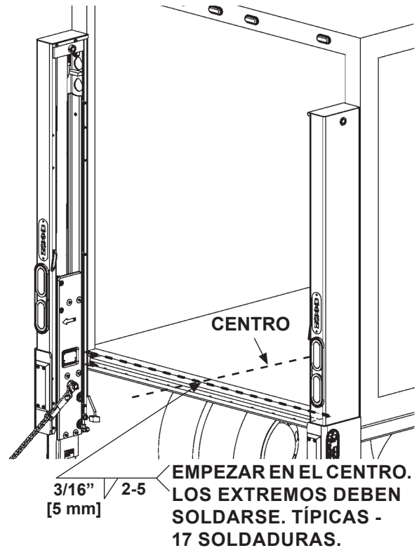
SOLDAR PARTE SUPERIOR DE LA PLACA DE EXTENSIÓN FIG. 81-1
