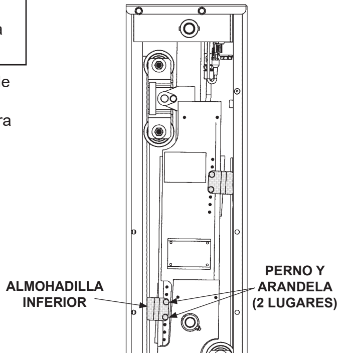
DESATORNILLAR LAS ALMOHADILLAS (SE MUESTRA LA COLUMNA Y CORREDERA IZQUIERDA) FIG. 87-2
