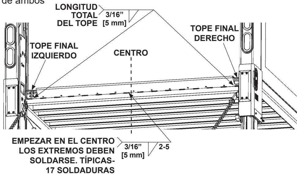
SOLDAR PARTE INFERIOR DE LA PLACA DE EXTENSIÓN FIG. 81-2
