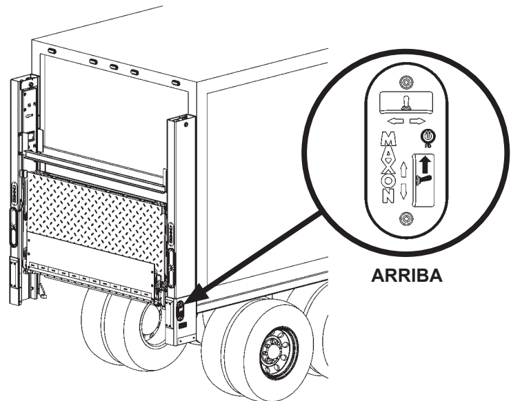
PRESURIZAR CILINDROS DE ELEVACIÓN FIG. 68-1
