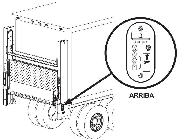
ELEVAR LA PLATAFORMA FIG. 72-2
