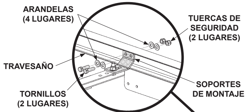
ATORNILLAR SOPORTES (8 LUGARES) FIG. 45-2A
