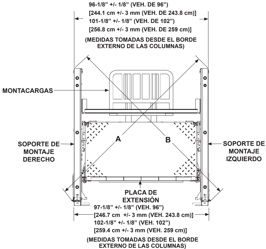
REVISAR SI LAS COLUMNAS ESTÁN EN CUADRO (SE MUESTRA PARTE POSTERIOR DEL ELEVADOR) FIG. 29-1
