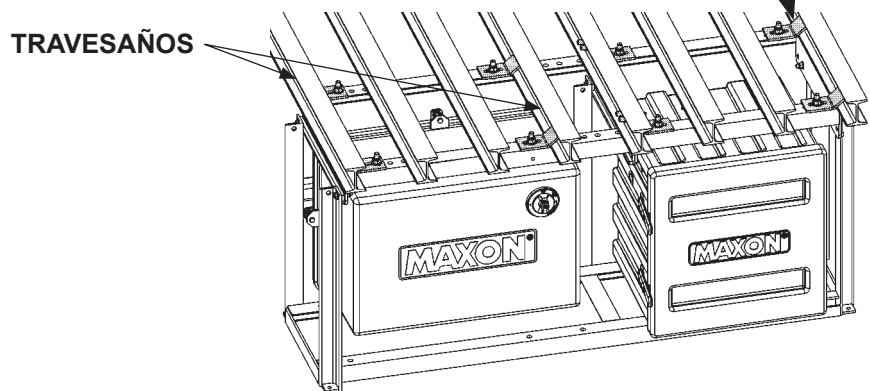
ATORNILLAR MARCO DE LA CAJA DE LA BATERÍA Y LA BOMBA FIG. 45-2
