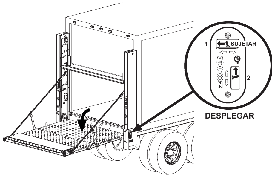
DESPLEGAR PLATAFORMA FIG. 69-2
