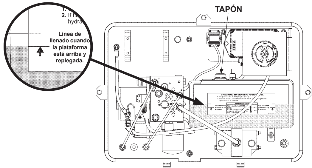
REVISAR EL NIVEL DEL FLUIDO HIDRÁULICO FIG. 73-1
