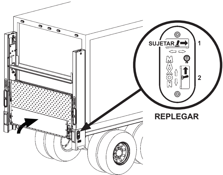
REPLEGAR LA PLATAFORMA FIG. 72-1
