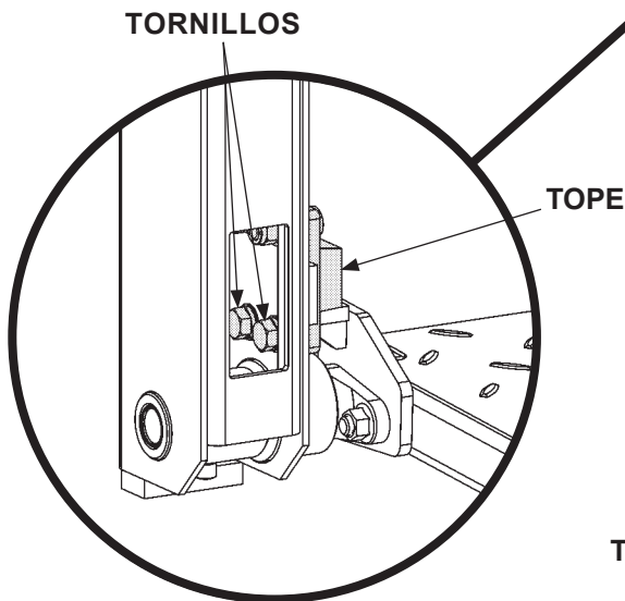
VISTA FRONTAL DE LA CORREDERA IZQUIERDA FIG. 84-1B
