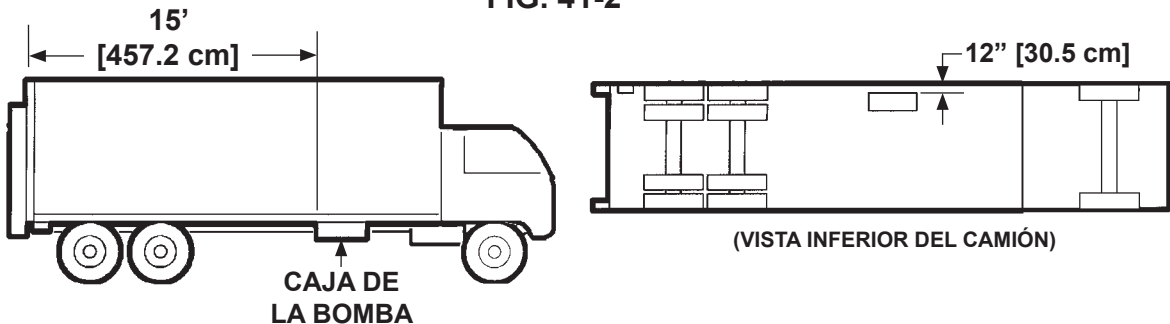
INSTALACIÓN USUAL PARA 15 PIES [457.2 cm] FIG. 41-3
