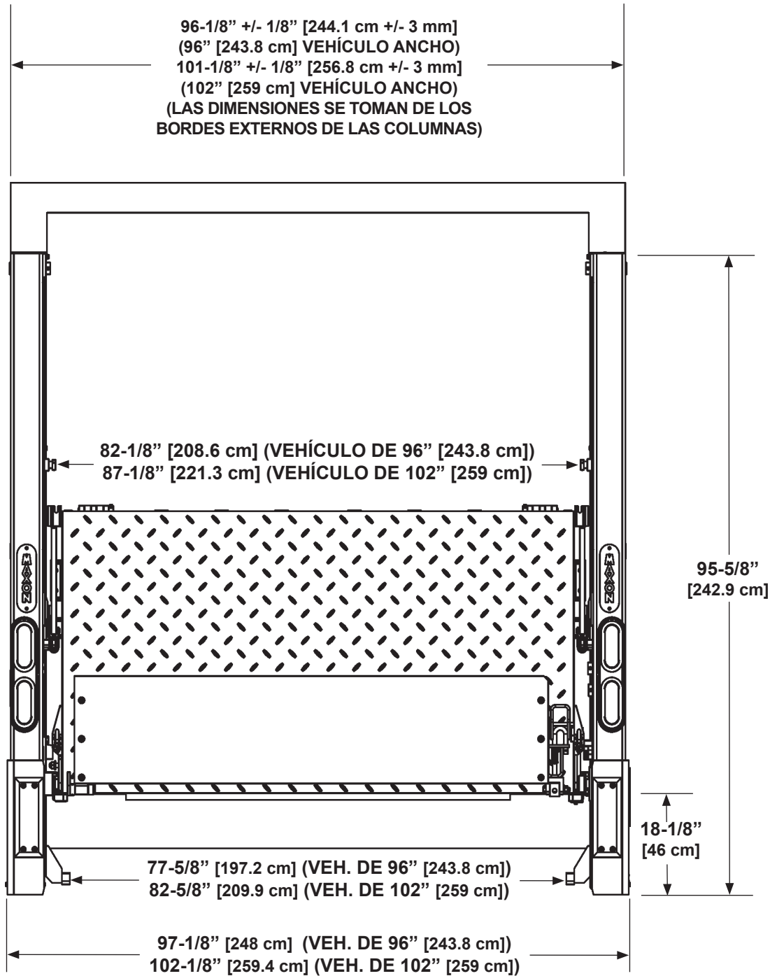
MEDIDAS DE MÁRGENES FIG. 11-1
