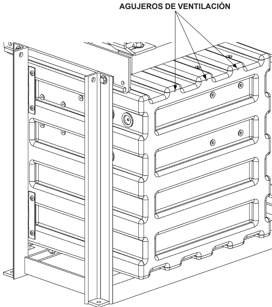
ENSAMBLE CAJA DE BATERÍA (SE MUESTRA LA VISTA POSTERIOR) FIG. 48-1
