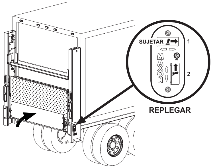
REPLEGAR PLATAFORMA FIG. 70-1
