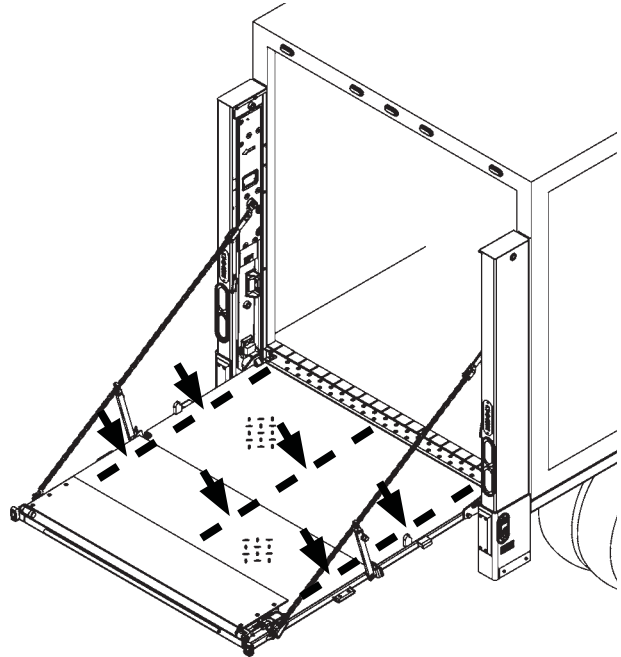
LAS FLECHAS INDICAN DÓNDE REVISAR SI LA PLATAFORMA Y LA PLATAFORMA ABATIBLE ESTÁN AL NIVEL
