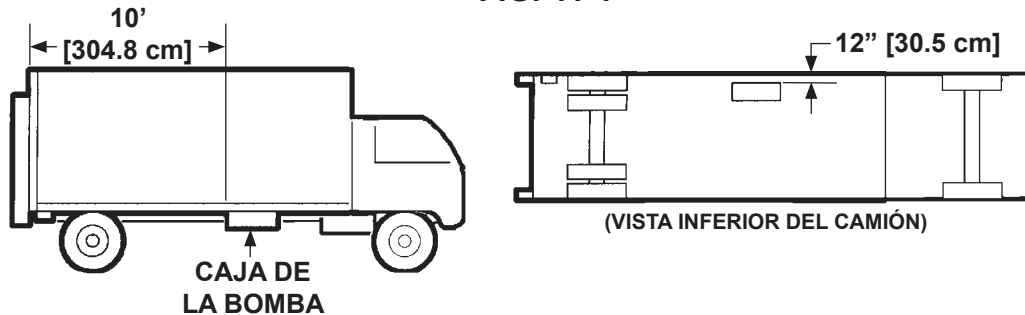
INSTALACIÓN USUAL PARA 10 PIES [304 cm] FIG. 41-2
