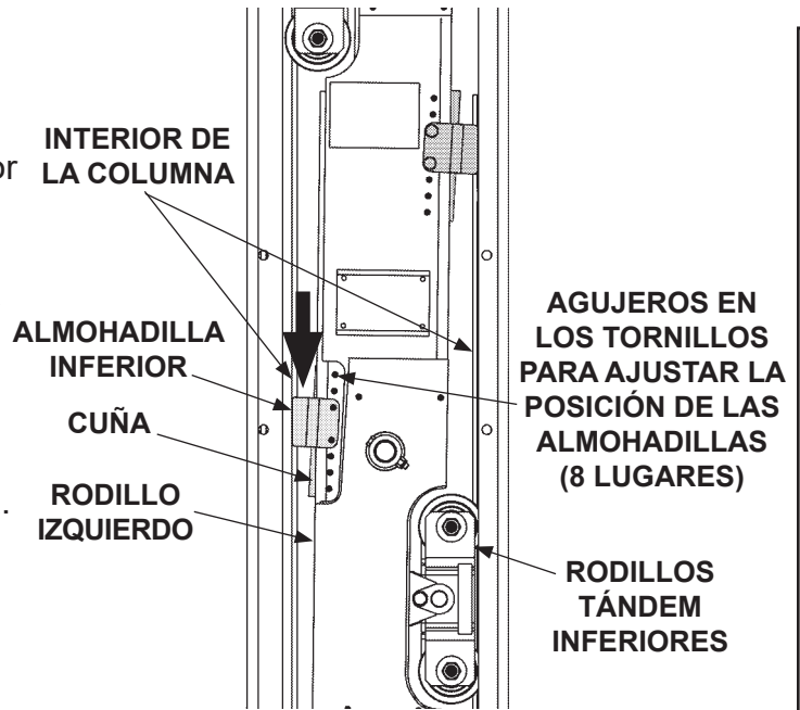
AJUSTAR LA ALMOHADILLA INFERIOR FIG. 88-1
