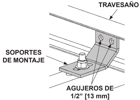
MARCAR Y TALADRAR FIG. 45-1
