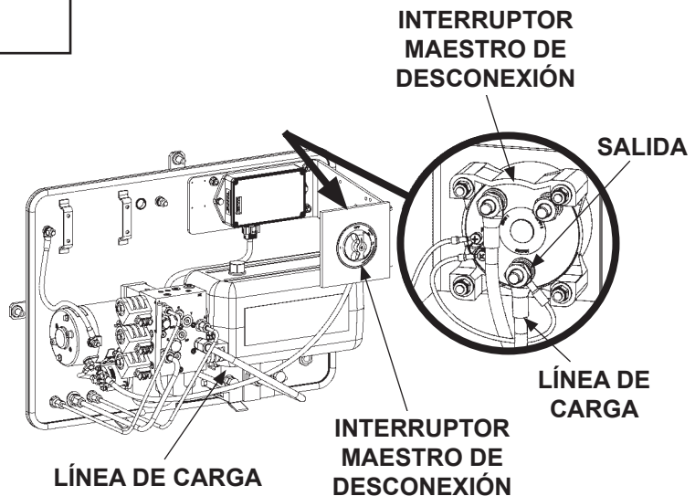
CONECTAR LÍNEA DE CARGA AL INTERRUPTOR MAESTRO DE DESCONEXIÓN FIG. 64-2
