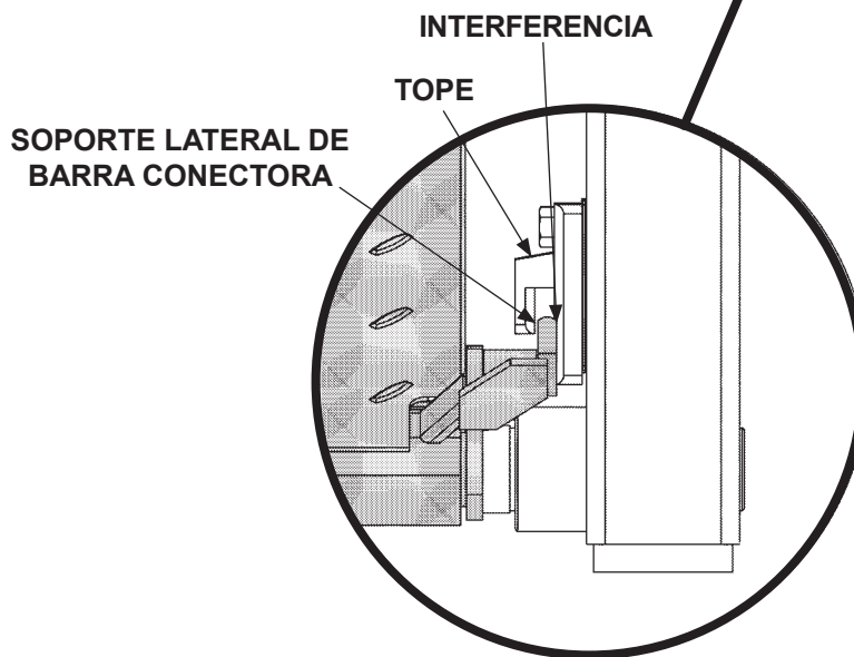
VISTA POSTERIOR DE CORREDERA IZQUIERDA FIG. 83-1A
