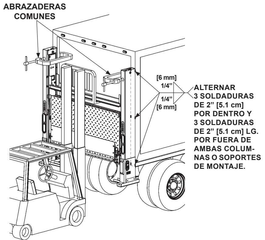
SOLDAR ELEVADOR AL VEHÍCULO FIG. 34-1
