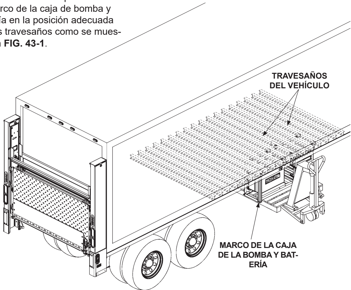
TRÁILER CON MARCO DE CAJA DE BOMBA Y BATERÍA FIG. 43-1
