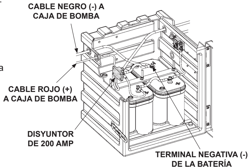
CONEXIONES ELÉCTRICAS EN LA CAJA DE BATERÍA FIG. 66-2
