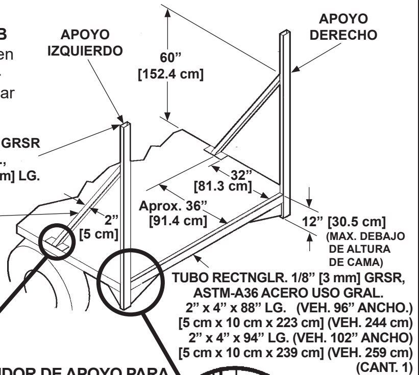
BASTIDOR DE APOYO PARA ELEVADOR EN PLATAFORMA FIG. 19-1A
