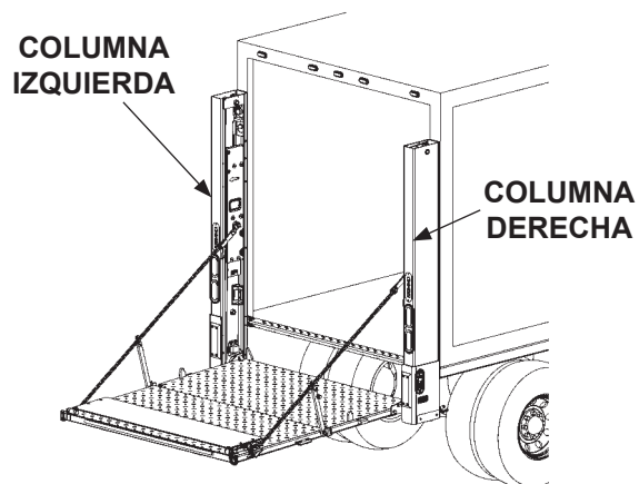
REVISAR EL ESPACIO ENTRE LAS ALMOHADILLAS CON LA PLATAFORMA ENTRE EL NIVEL DE CAMA Y EL SUELO FIG. 86-2
