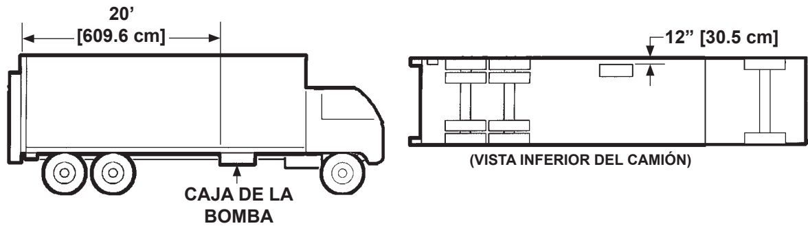
INSTALACIÓN USUAL PARA 20 PIES [609.6 cm] FIG. 42-1
