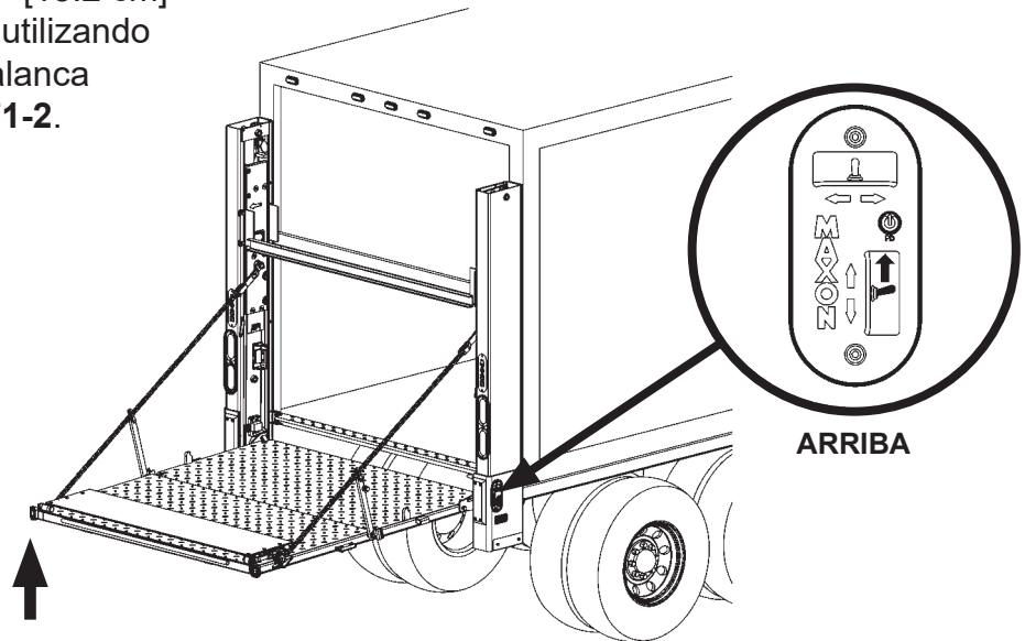
ELEVAR LA PLATAFORMA FIG. 71-2
