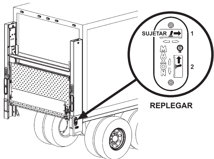
PRESURIZAR CILINDRO DE CIERRE FIG. 68-2
