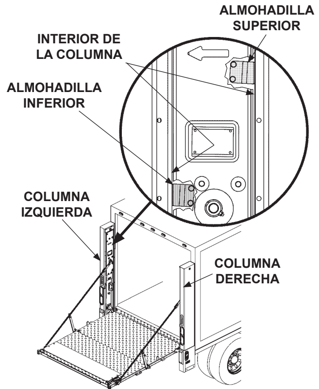
REVISAR EL ESPACIO ENTRE LAS ALMOHADILLAS CON LA PLATAFORMA AL NIVEL DE CAMA FIG. 86-1
