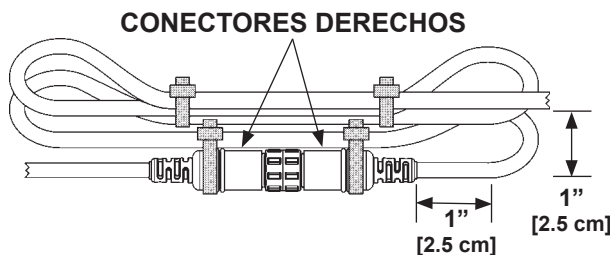
ALINEAMIENTO CORRECTO DEL CABLE FIG. 57-2
