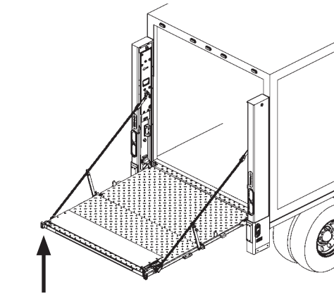
PLATAFORMA AL NIVEL DE CAMA FIG. 85-1
