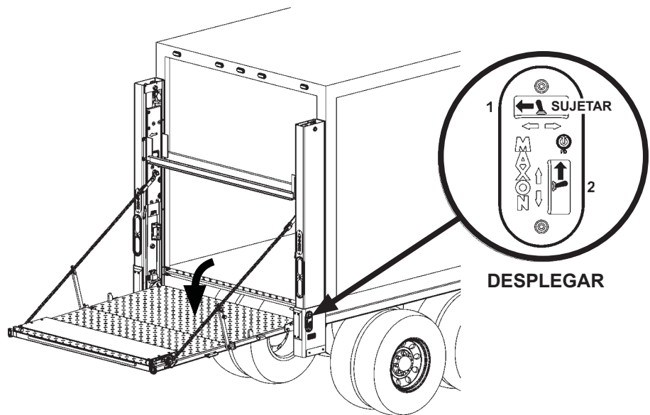
DESPLEGAR PLATAFORMA FIG. 70-2
