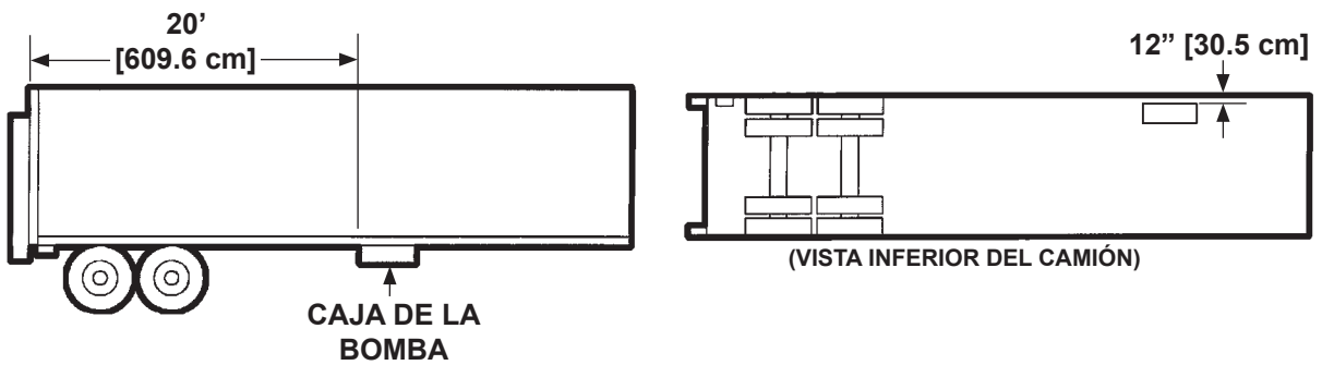
INSTALACIÓN USUAL PARA 20 PIES [609.6 cm] FIG. 42-2
