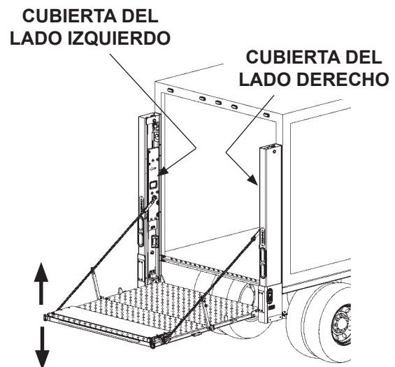
REVISAR EL ESPACIO ENTRE LAS ALMOHADILLAS CON LA PLATAFORMA ENTRE EL NIVEL DE CAMA Y EL SUELO FIG. 89-2
