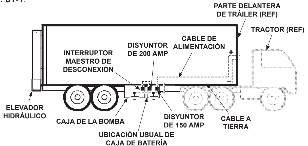
INSTALACIÓN RECOMENDADA DEL ELEVADOR Y LA CAJA DE BATERÍA EN TRÁILER
