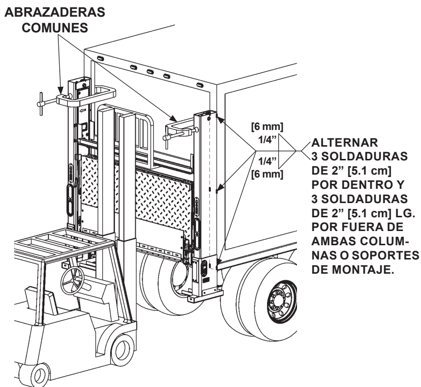
SOLDAR ELEVADOR AL VEHÍCULO FIG. 30-1
