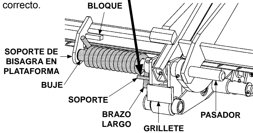
INSTALAR EL PASADOR DE BISAGRA (SE MUESTRA LADO DERECHO DE PLATAFORMA) FIG. 19-1
