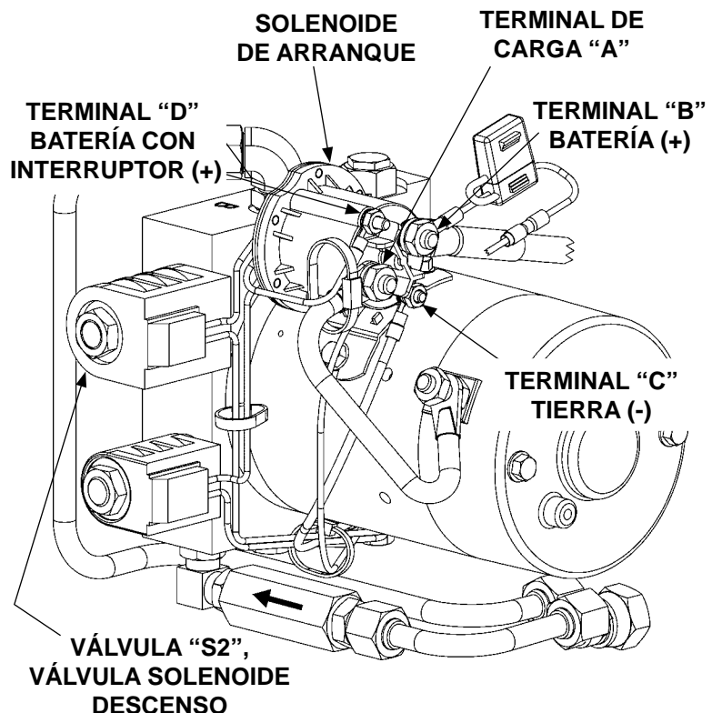
UNIDAD DE PODER DESCENSO ASISTIDO
