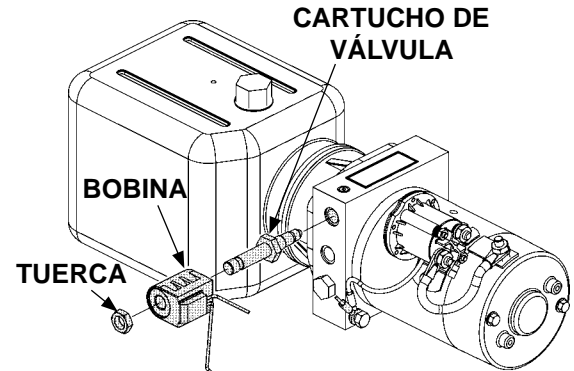
REMOVER VÁLVULA DE SOLENOIDE (UNIDAD DE PODER DESCENSO POR GRAVEDAD) FIG. 41-1
