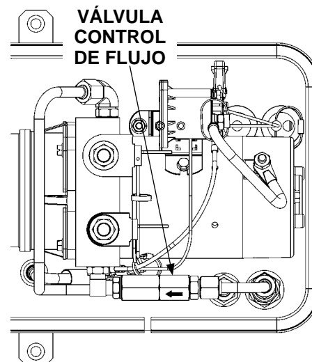
VÁLVULA CONTROL DE FLUJO EN PARTE POSTERIOR DEL ENSAMBLAJE DE LA BOMBA CON DESCENSO ASISTIDO FIG. 47-2
