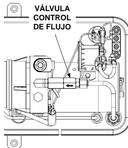
VÁLVULA CONTROL DE FLUJO EN PARTE POSTERIOR DEL ENSAMBLAJE DE LA BOMBA CON DESCENSO POR GRAVEDAD FIG. 47-1
