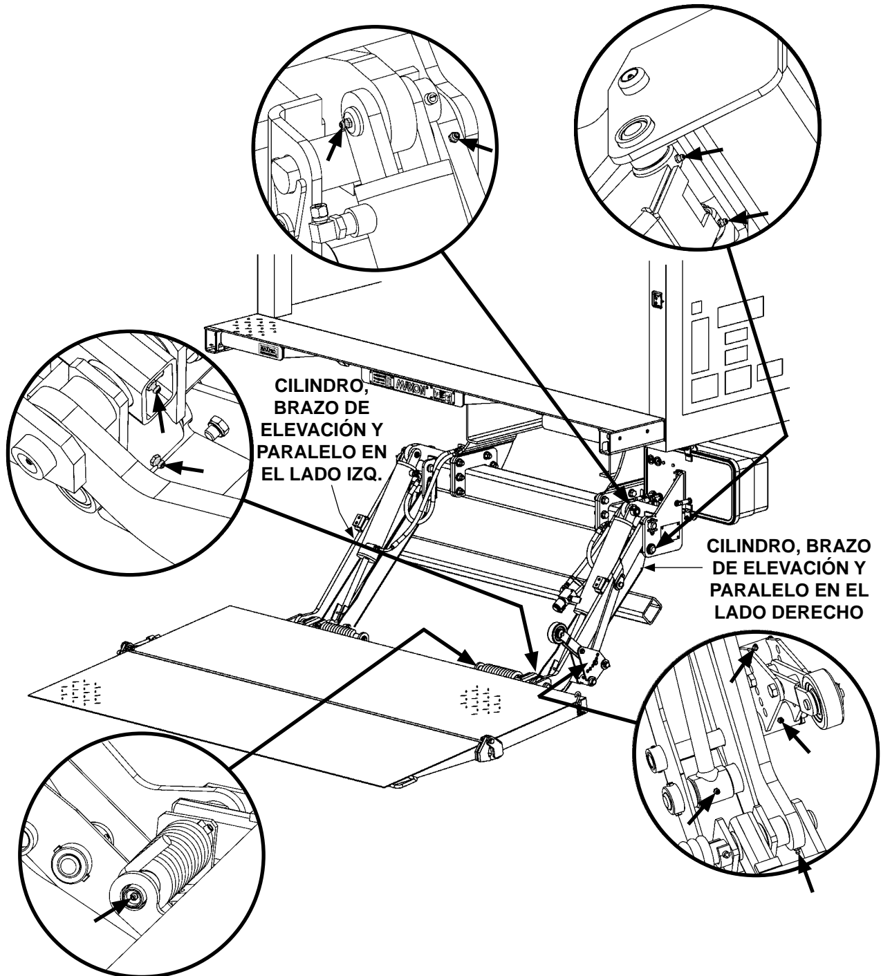
DIAGRAMA DE LUBRICACIÓN TE-33 FIG. 13-1
