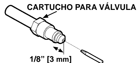
REVISAR VÁLVULA DE SOLENOIDE FIG. 47-3
