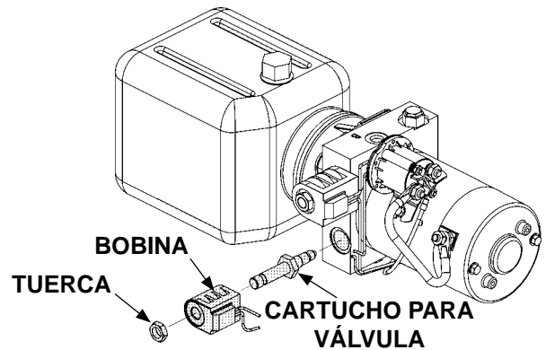
REMOVER VÁLVULA DE SOLENOIDE (UNIDAD DE PODER DESCENSO ASISTIDO) FIG. 41-2
