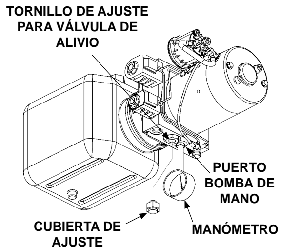
AJUSTAR LA VÁLVULA DE ALIVIO DE ELEVACIÓN (UNIDAD DE PODER DESCENSO ASISTIDO) FIG. 44-2
