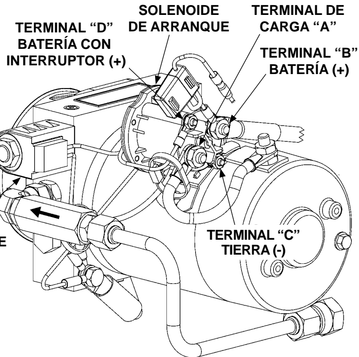
UNIDAD DE PODER DESCENSO POR GRAVEDAD
