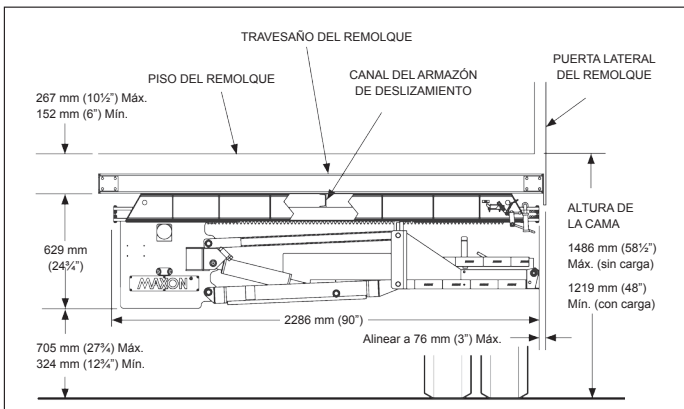
Dimensiones y requisitos de montaje del liftgate
